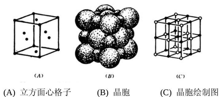
图 1 氯化钠晶体结构
