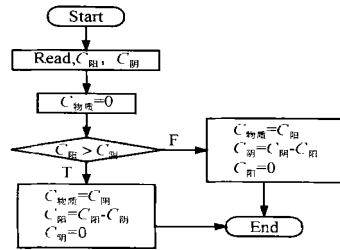
图 4 Select 子程序流程
