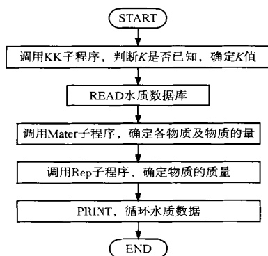
图 1 主程序流程
