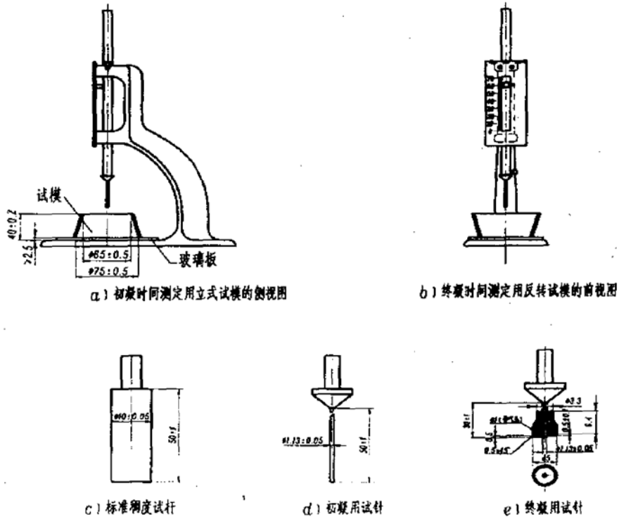
图 1 测定水泥标准稠度和凝结时间用的维卡仪
